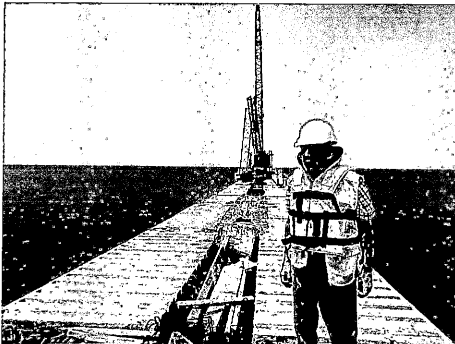
SUPERVISOR EN EJE 171, LA GRUA Y MARTILLO EN EJE 177
