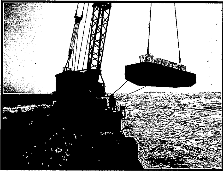
07.04.07.07 COLOCACION DE VIGAS TRANSVERSALES DEL EJE 170 AL 177.
