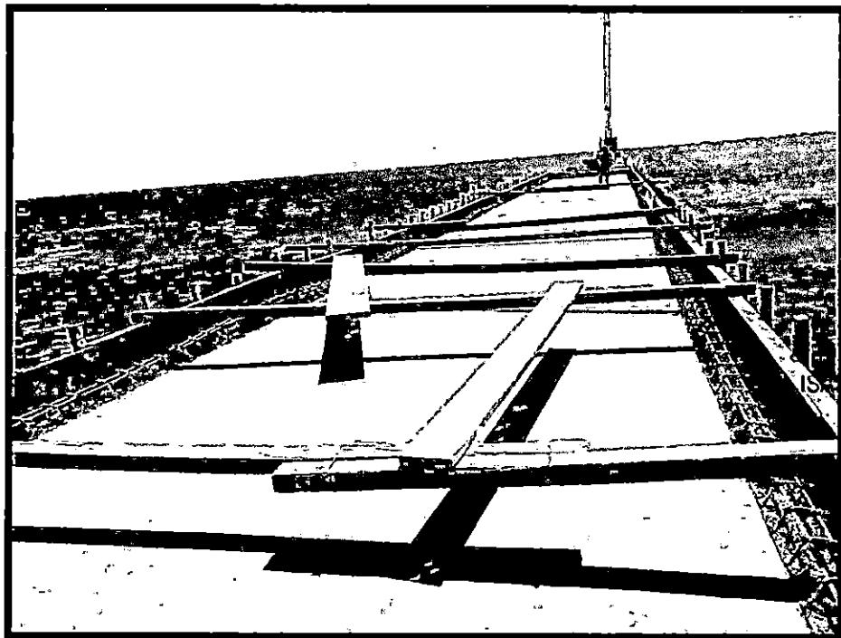
Concreto en Losa (Eje 136 al 151)
